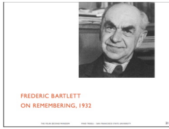
trogu / 4-second - 21
