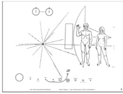
trogu / 4-second - 08
